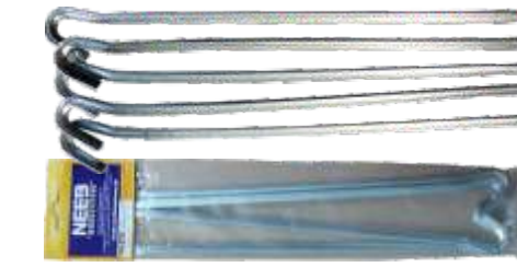
Set Spezial-Erdnägeln (VE = 5 Stück) Artikel-Nr.: S220009
