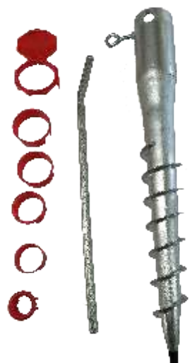
Bodendübel Artikel-Nr.: S220009
